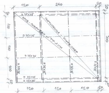
ОСНОВА КРОВА /ШЕНА КОНСТРУКЦИЈЕ/
